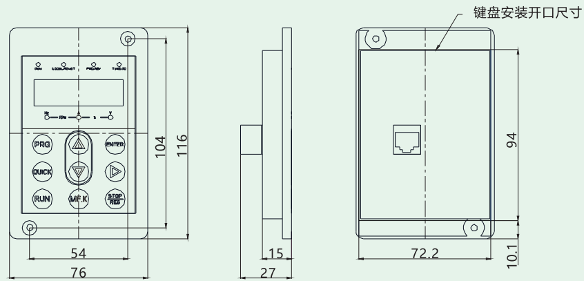
键盘尺寸图 (mm)
