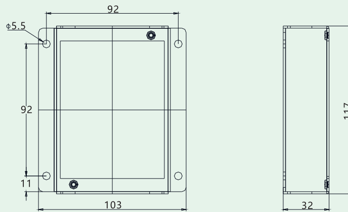
键盘托架尺寸图 (mm)
