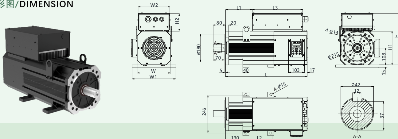
HY02一体机 18系列规格型号及额定参数 Specifications, models and rated parameters
