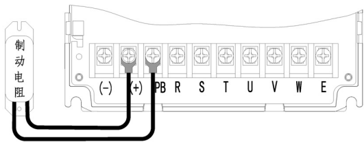
图 3-10：SD650 系列伺服驱动器 110KW（含）以下机器制动电阻的连接图
