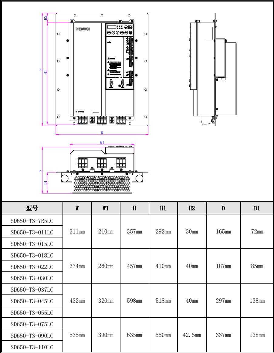
图 3-2：SD650 液冷 (LC) 系列伺服驱动器外形结构尺寸图
