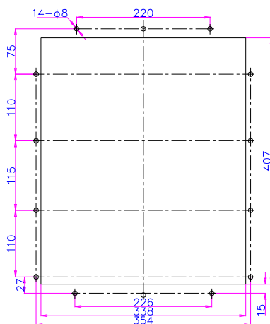
18.5KW-30KW安装固定开孔图
