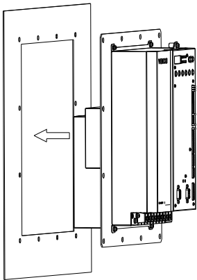
图 3-3：SD650 液冷 (LC) 系列伺服驱动器的安装固定开孔图
