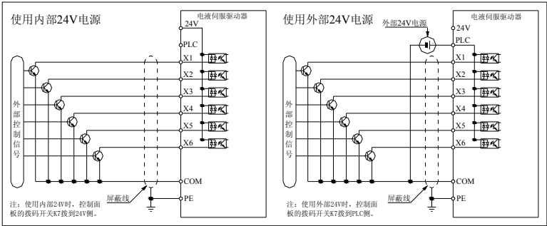
图 3-8：NPN 特性晶体管的多功能输入信号连接方式
