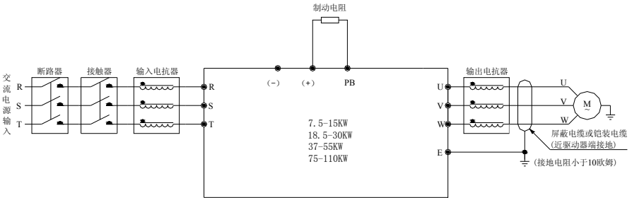
图 3-6：SD650 系列伺服驱动器主回路接线图
