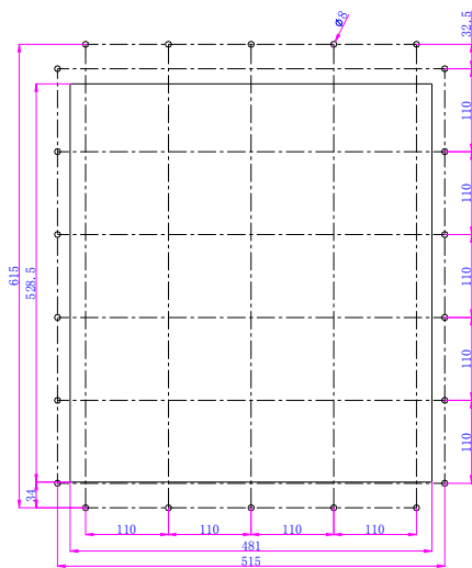
75KW-110KW 安装固定开孔图
