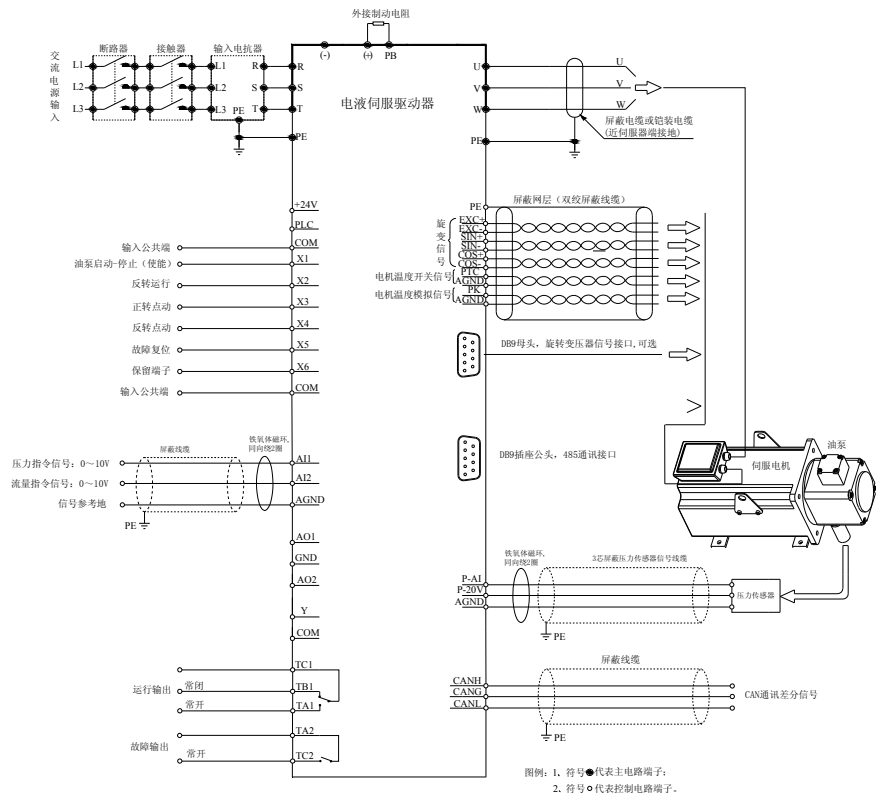
图 3-5：SD650 系列伺服驱动器接线图
