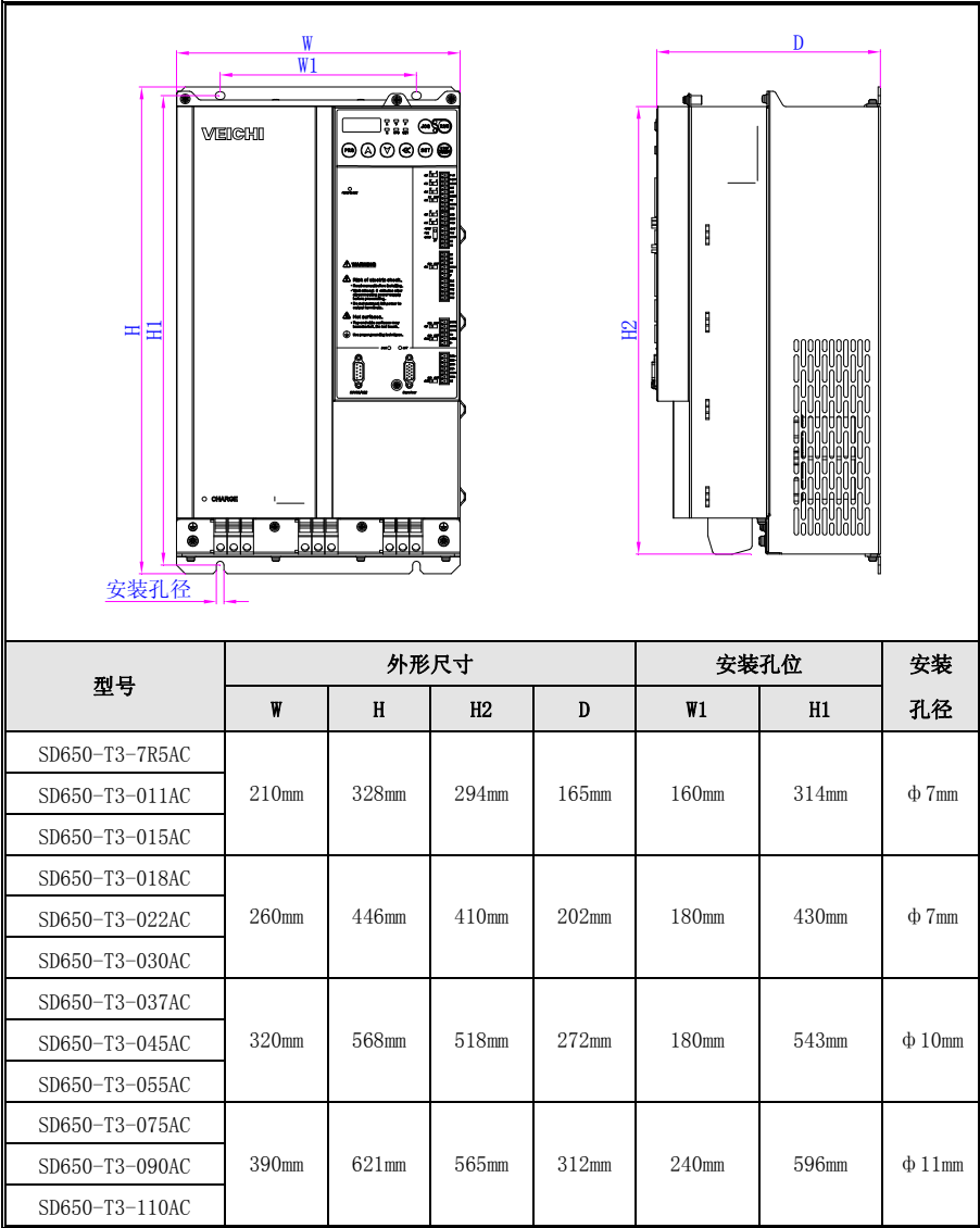
图 3-1：SD650 风冷 (AC) 系列伺服驱动器外形结构尺寸图
