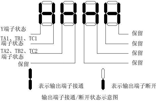
输出端子断开接通状态示意图：
