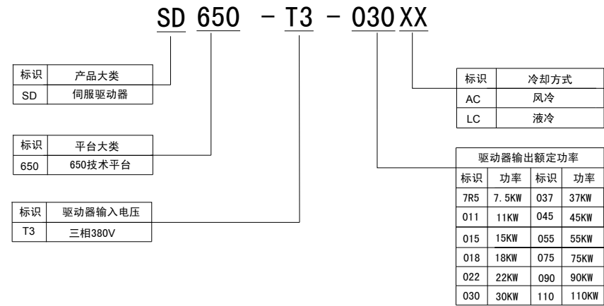
图 2-2：SD650 系列伺服驱动器铭牌含义及命名规则
