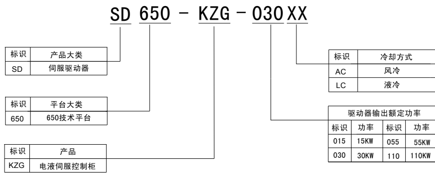
图 2-3：SD650 系列控制柜铭牌含义及命名规则
