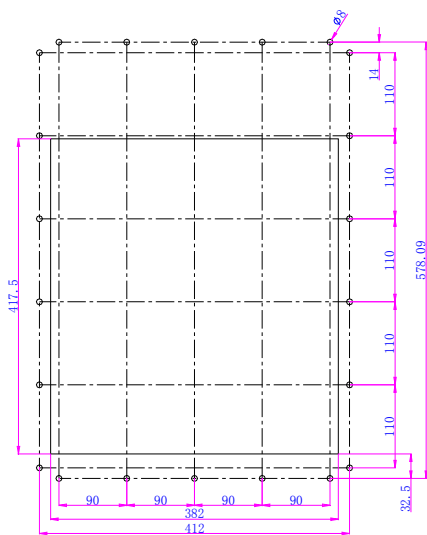
37KW-55KW 安装固定开孔图
