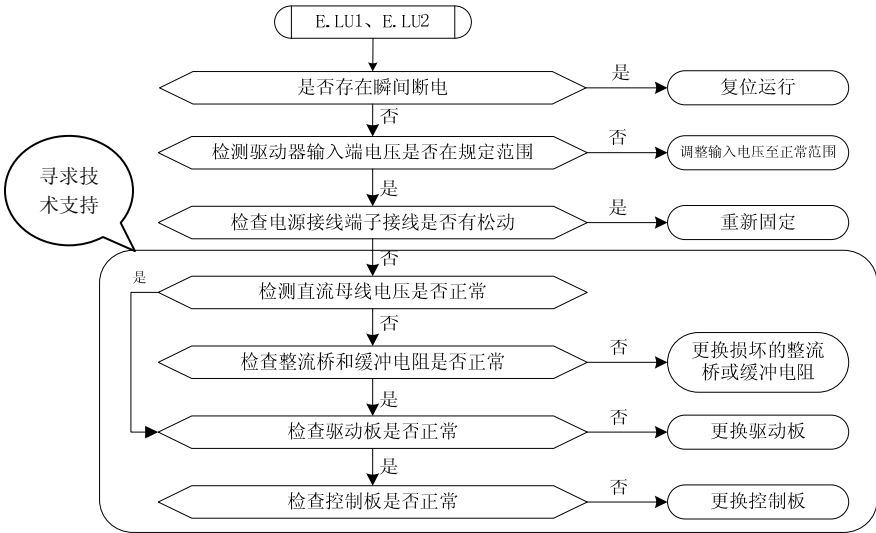
驱动器欠压故障(E.LU1、E.LU2)
