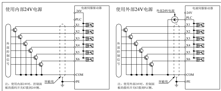
图 3-8：NPN 特性晶体的多功能输入信号连接方式
