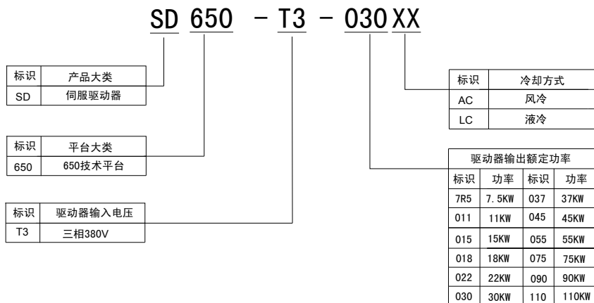
图 2-2：SD650 系列伺服驱动器铭牌含义及命名规则
