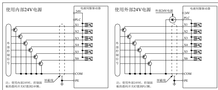
图 3-9：PNP 特性晶体的多功能输入信号连接方式
