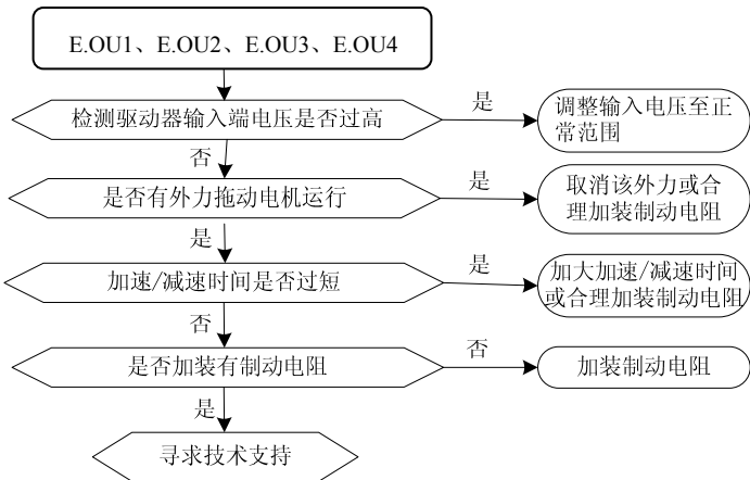
驱动器过压故障(E.OU1、E.OU2、E.OU3、E.OU4)
