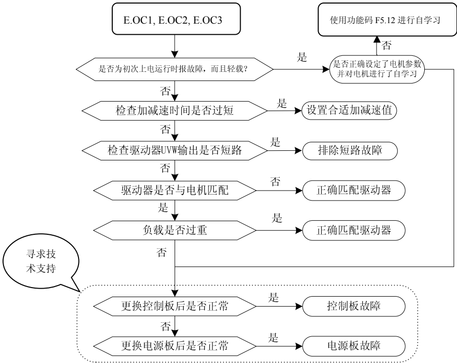
过流故障 (E. OC1, E. OC2, E. OC3)
