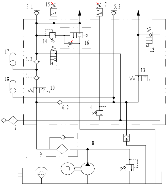
液压制动系统实例丹麦 BONUS-150KW 风机刹车液压系统
